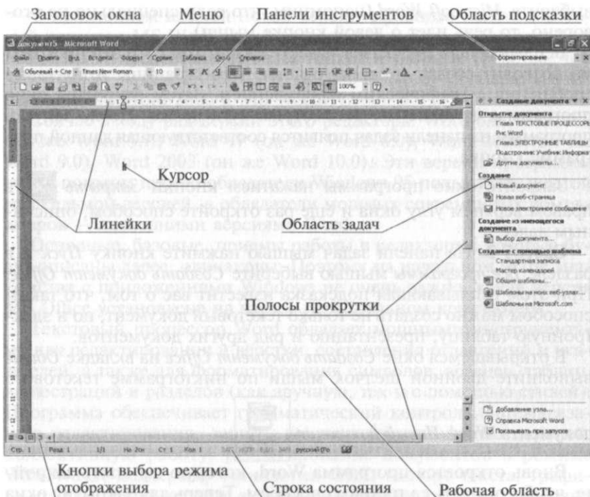
Рис. 10.1. Общий вид окна программы MS Word
