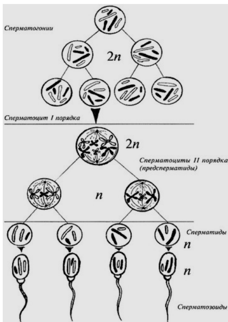
Рис. 1. Схема сперматогенеза
